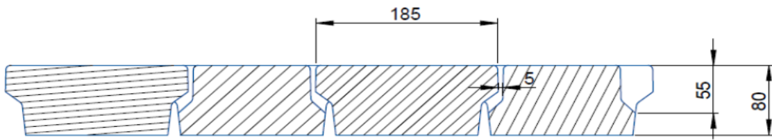
COUPE B-B
