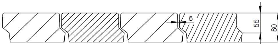
COUPE B-B
